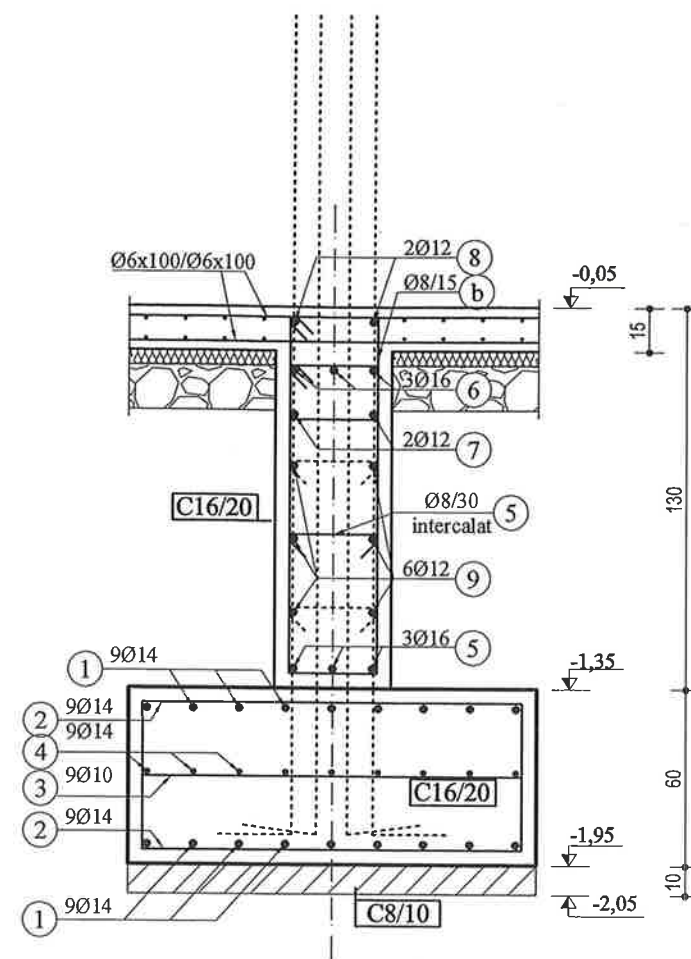
Fundatie F1 -interior-
