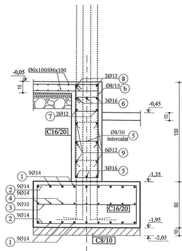
Fundatie F1 -exterior-
